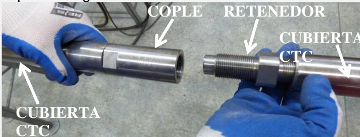
Cable ACCEC® + Cubierta CTC + Cople CTC mediano + Cubierta CTC + Cable ACCEC®
